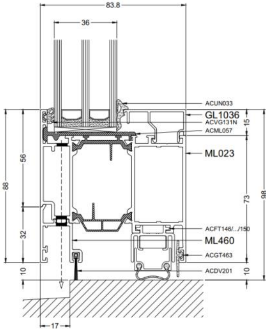
Les traverses dans l'ouvrant de porte.
